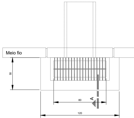
PLANTA BAIXA
