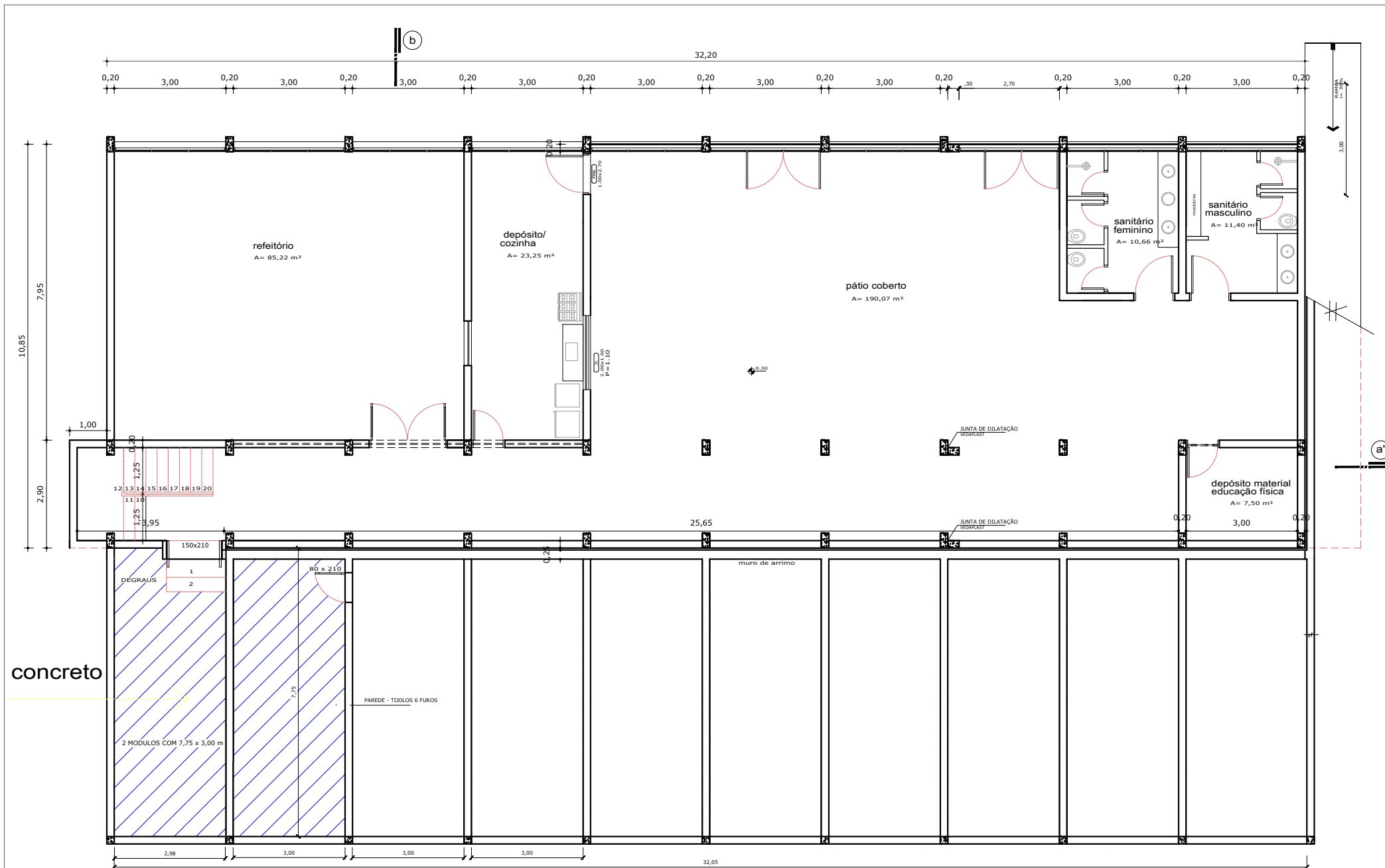
planta baixa pav. inferior A= 238,40 m²
