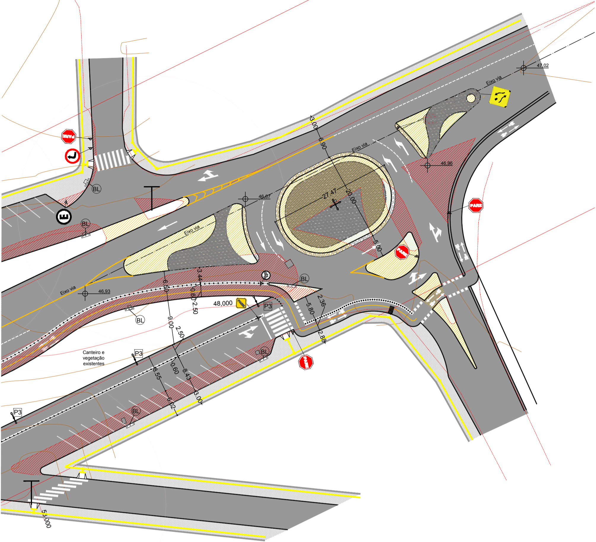
PLANTA DE PAVIMENTAÇÃO H esc. 1:500
