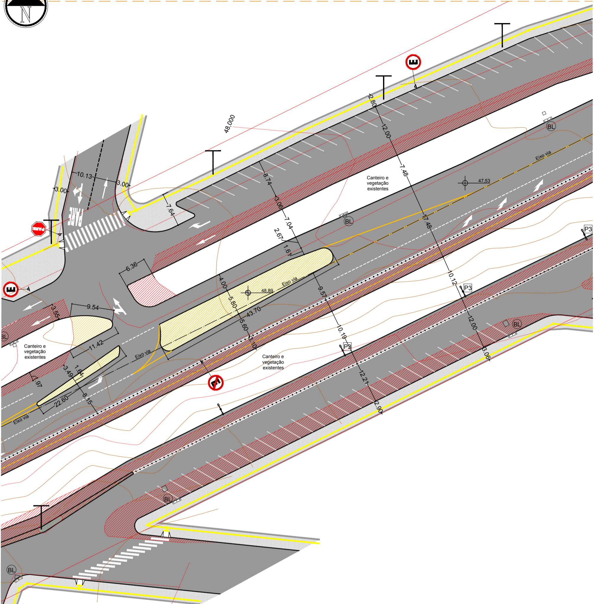
PLANTA DE PAVIMENTAÇÃO G esc. 1:500
