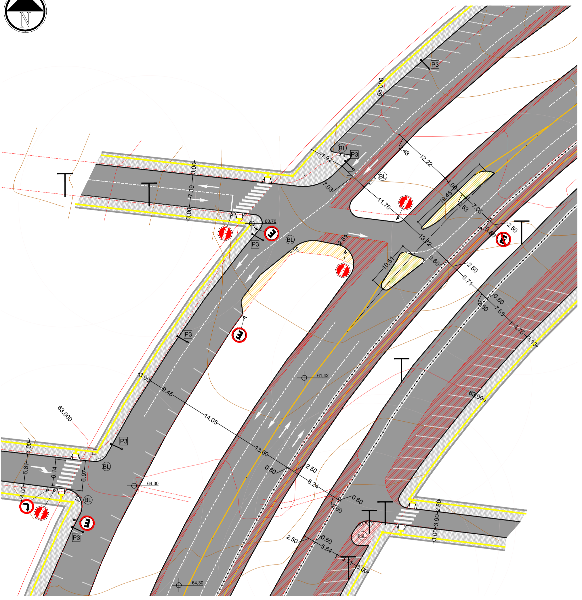
PLANTA DE PAVIMENTAÇÃO E esc. 1:500
