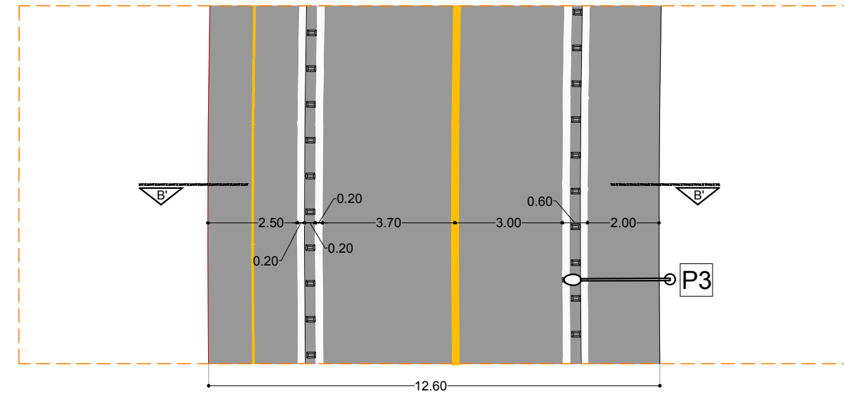
SETOR DE PLANTA B'B'' esc. 1:150
