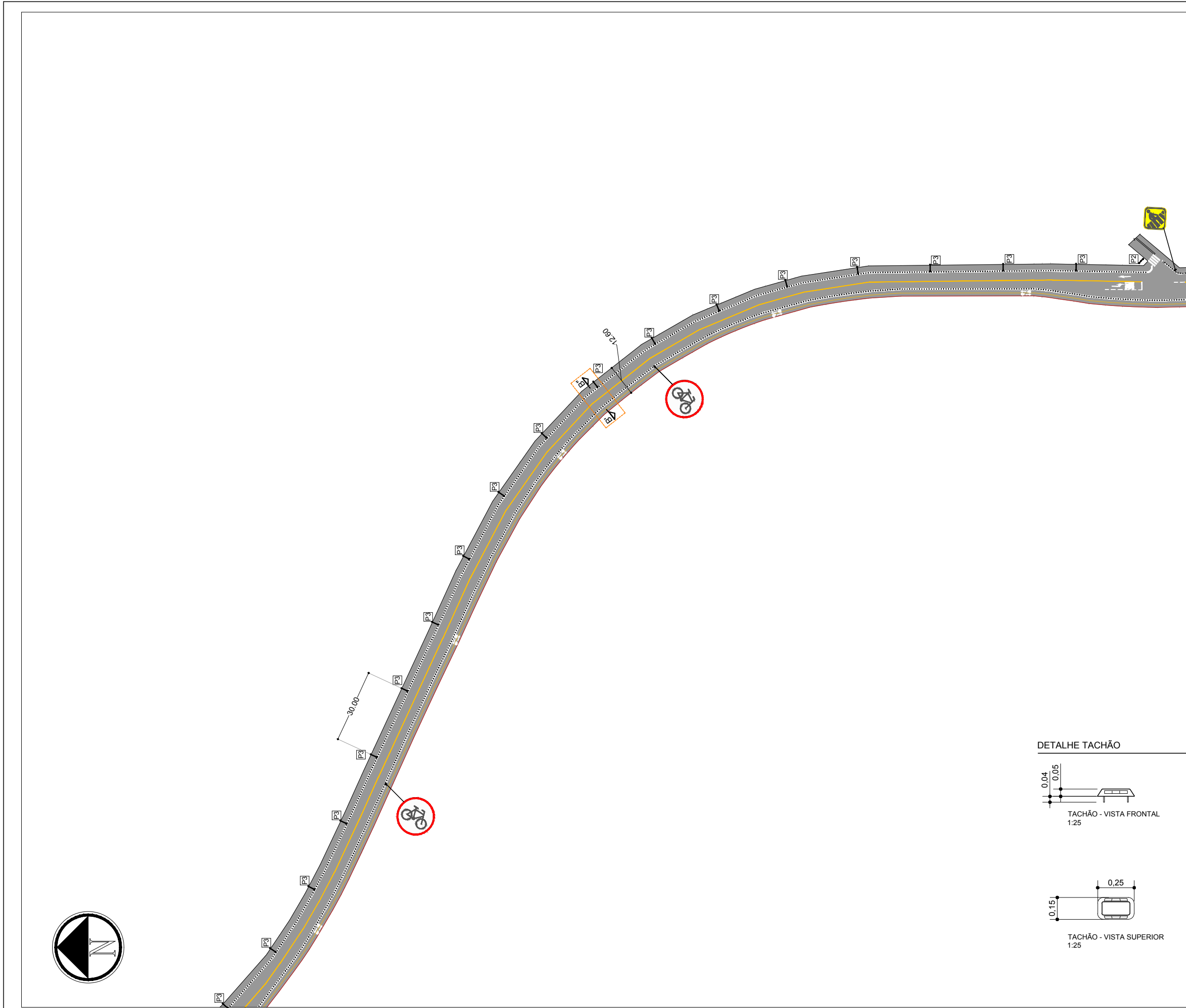
PLANTA DE PAVIMENTAÇÃO B esc. 1:1000
